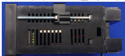
取付具（左右のネジで盤に挟み込み固定）
